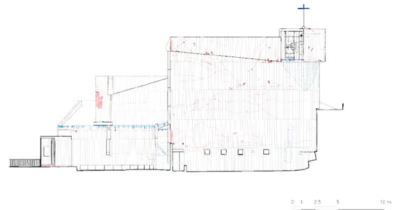
Figura 51: Levantamiento crítico fachadas norte, poniente y sur de la Iglesia del Monasterio de los Benedictinos.
