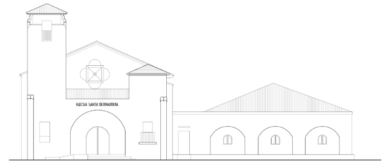
Figura 33: Elevación fachada norte Iglesia Santa Bernardita y sede social Vista Hermosa, 2022.
